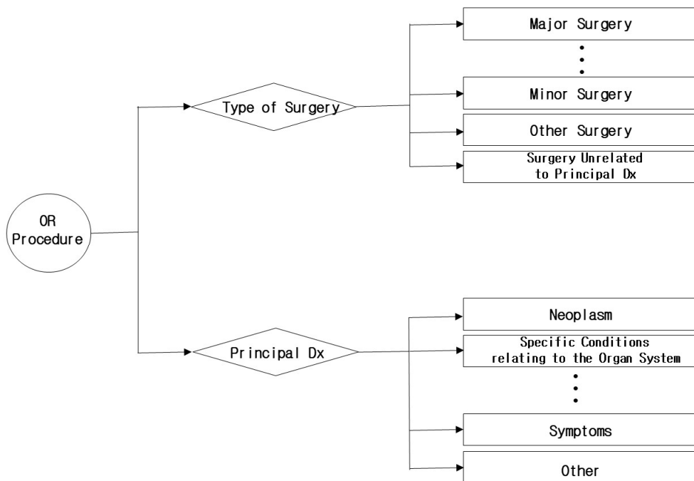
그림 2. ADRG 분류
